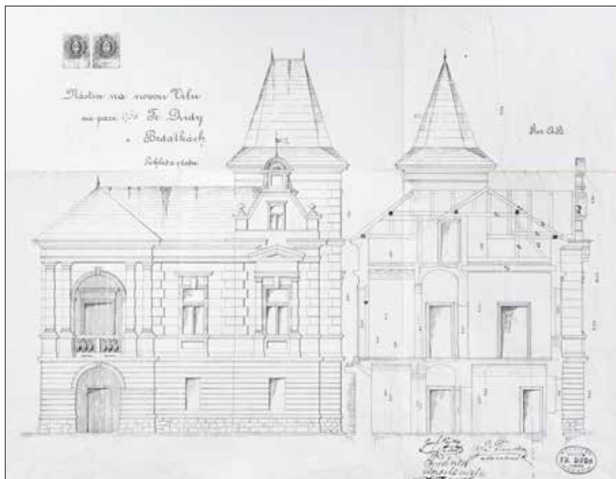
■ Výkres pro stavební povolení původní Dudovy vily. (Osobní archiv Michala Dejmal)
